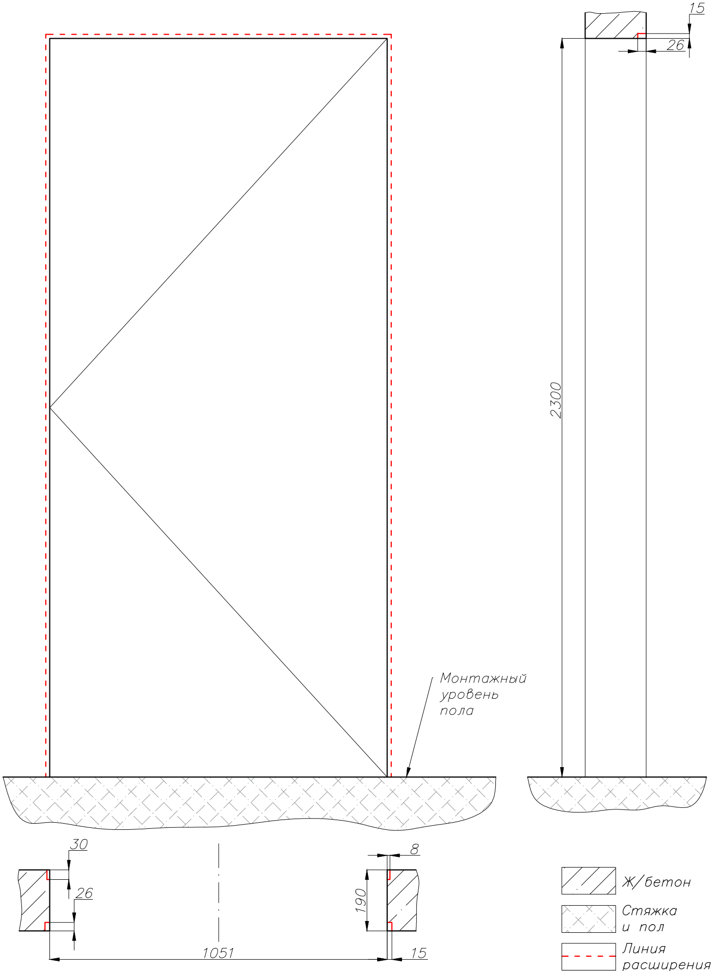
Вертикальный разрез
